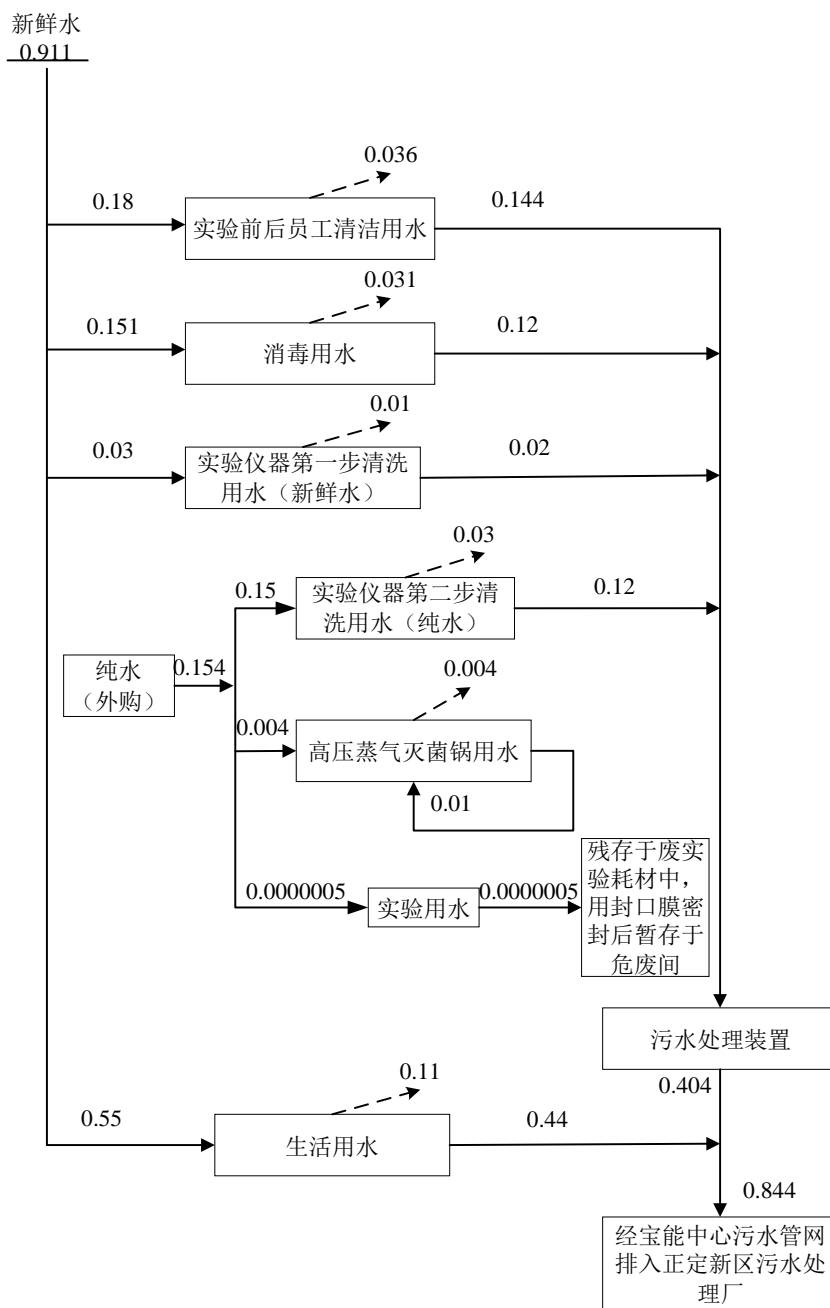
图 2-1 项目完成后全厂水平衡图 单位: m 3 /d
