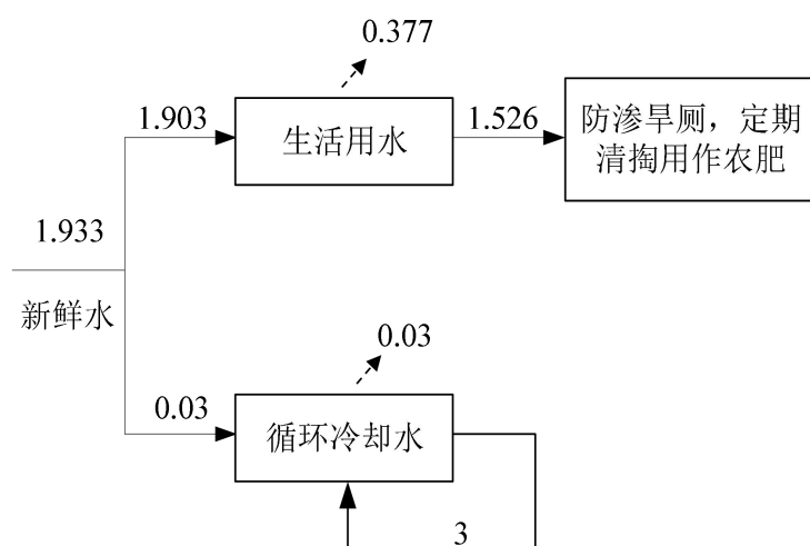
图 2 改扩建完成后全厂水平衡图 单位 \text{m}^3/\text{d}
