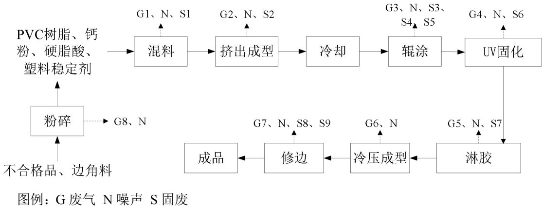
图2 项目 SPC 蜂窝板生产工艺流程及排污节点图
