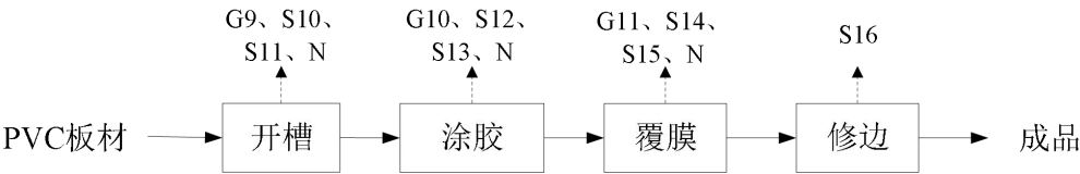
图3 项目环保装饰板材生产工艺流程及排污节点图
