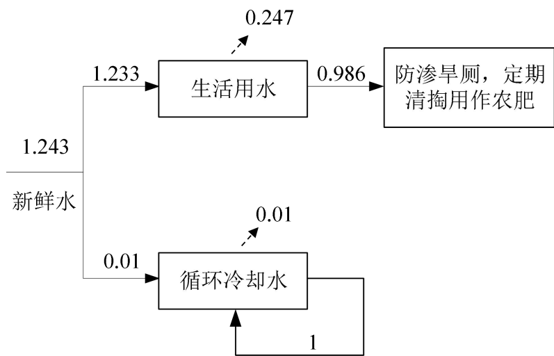
图 1 改扩建项目水平衡图 单位 m 3 /d
